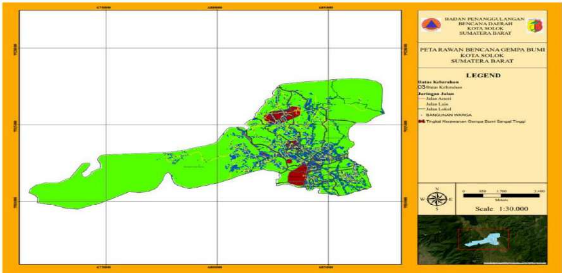
Gambar 2.26 Proyeksi Wilayah dan Penduduk Terdampak Bencana Gempa Bumi
